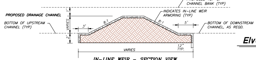
IN-LINE WEIR - SECTION VIEW N.T.S.
