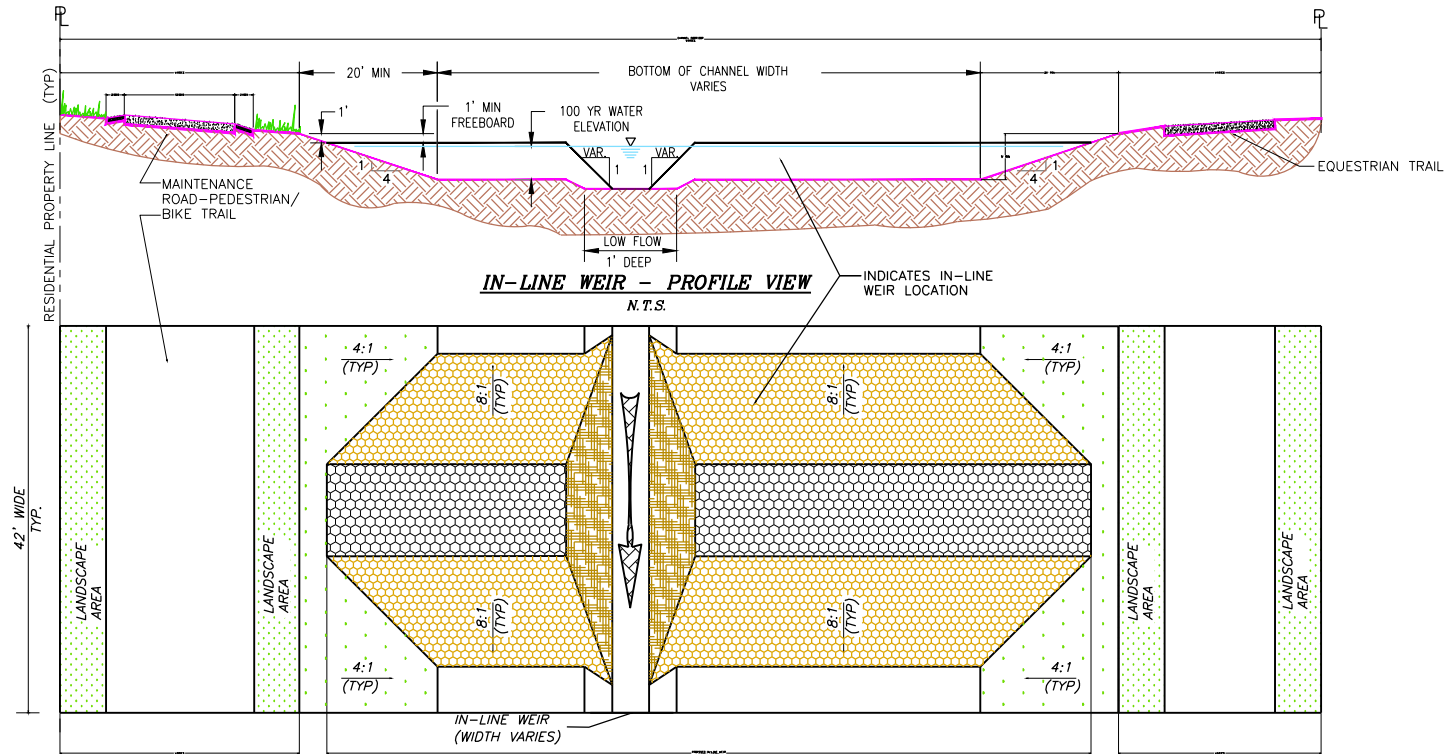
IN-LINE WEIR - PLAN VIEW N.T.S.
